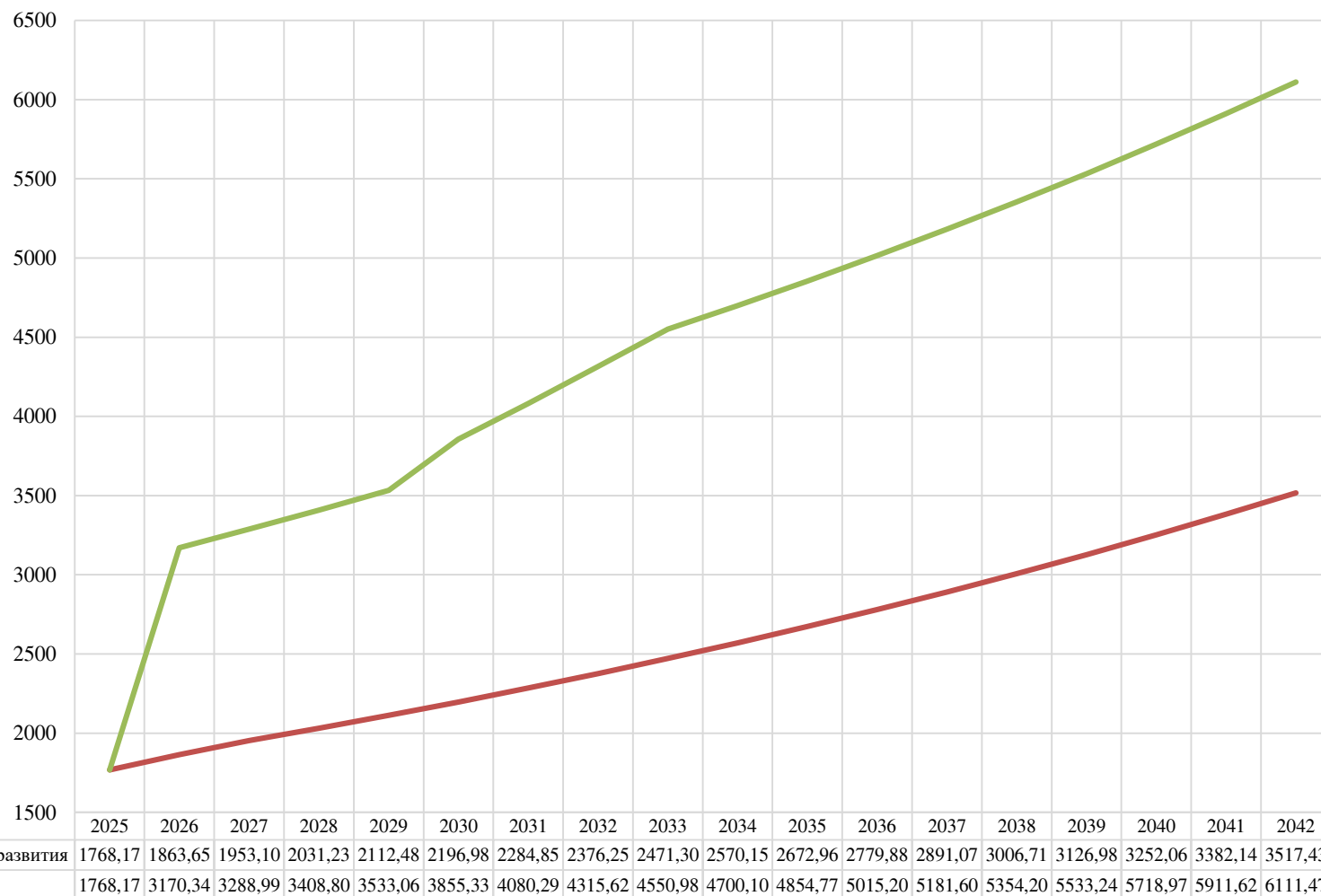
Рисунок 15.7 – Ценовые последствия для потребителей ЕТО №8 Негативные последствия по данной ЕТО связаны с избытком средств, выявленным по результатам анализа итогов ПХД за предшествующий период регулирования, а не с мероприятиями по развитию системы теплоснабжения. Данный фактор должен быть нивелирован при корректировке тарифа на тепловую энергию на 2026 г.
