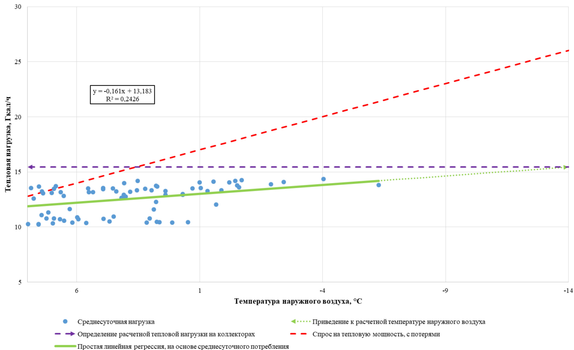
Рисунок 5.16 - Определение расчетной тепловой нагрузки на коллекторах в зоне действия котельной №1 ООО «Тепловик»
