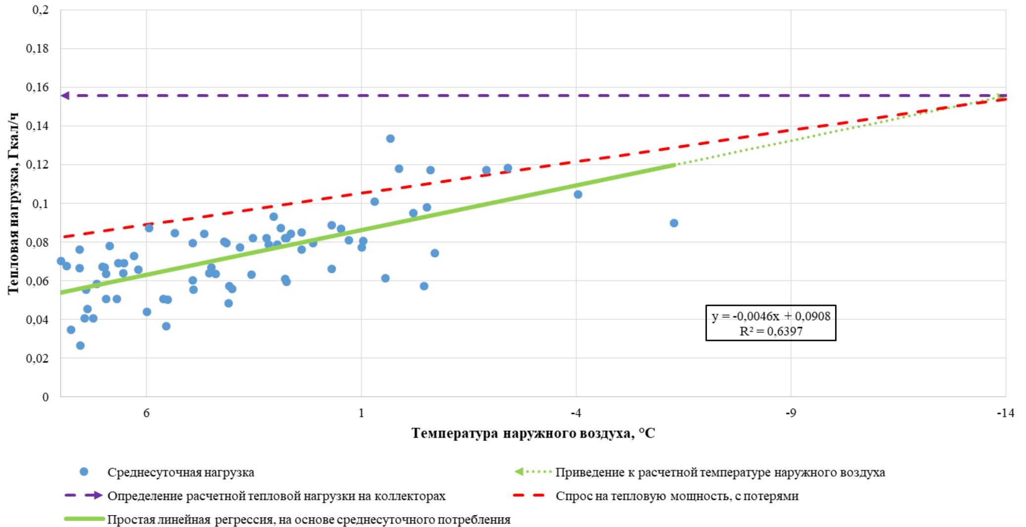
Рисунок 5.10 - Определение расчетной тепловой нагрузки на коллекторах в зоне действия котельной №11 АО «Теплоэнерго»
