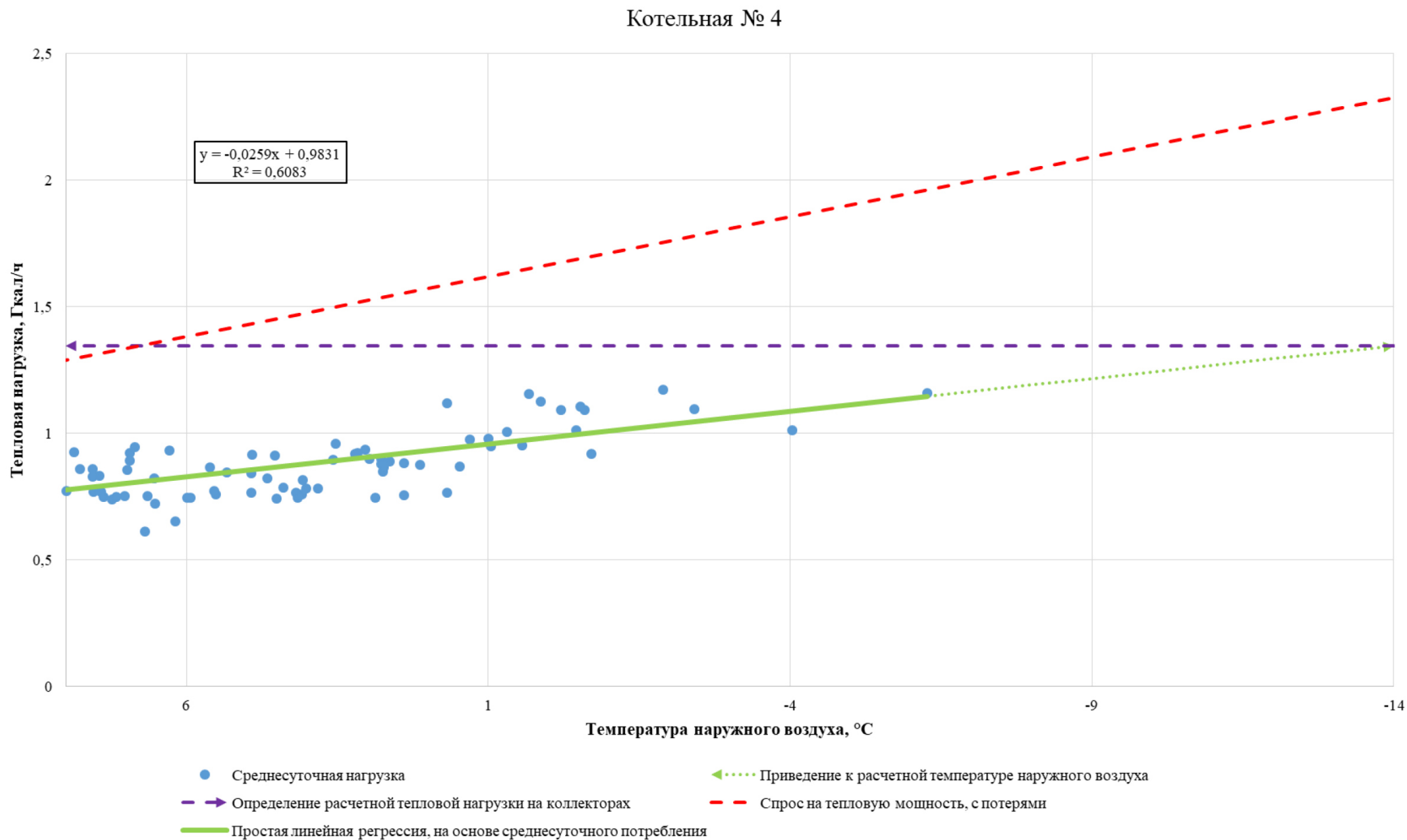
Рисунок 5.4 - Определение расчетной тепловой нагрузки на коллекторах в зоне действия котельной №4 АО «Теплоэнерго»
