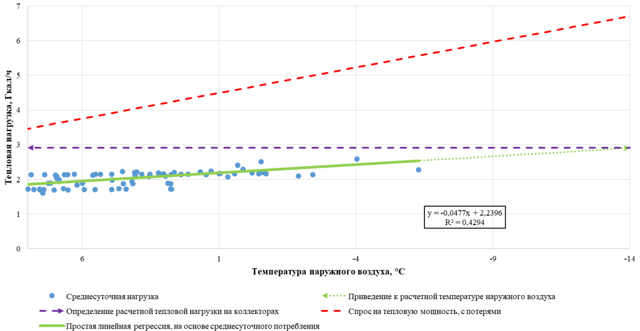
Рисунок 5.15 - Определение расчетной тепловой нагрузки на коллекторах в зоне действия котельной №23 АО «Теплоэнерго»
