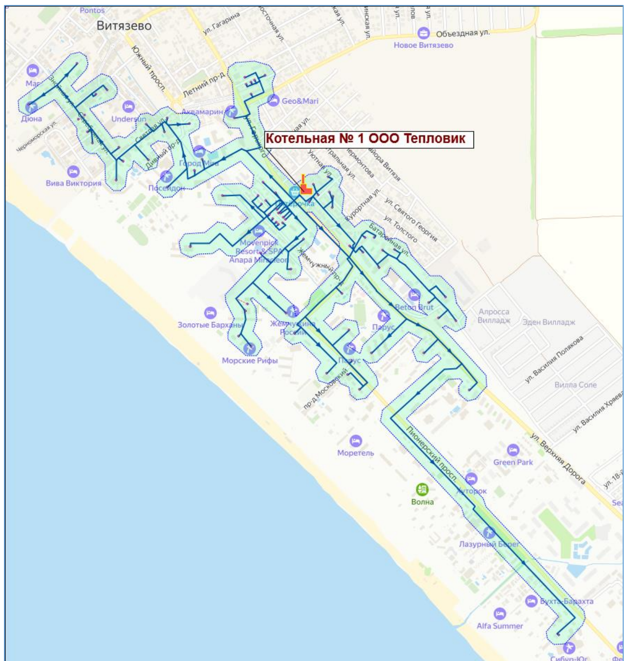
Рисунок 4.3 – Зона эксплуатационной ответственности котельной № 1 ООО «Тепловик»
