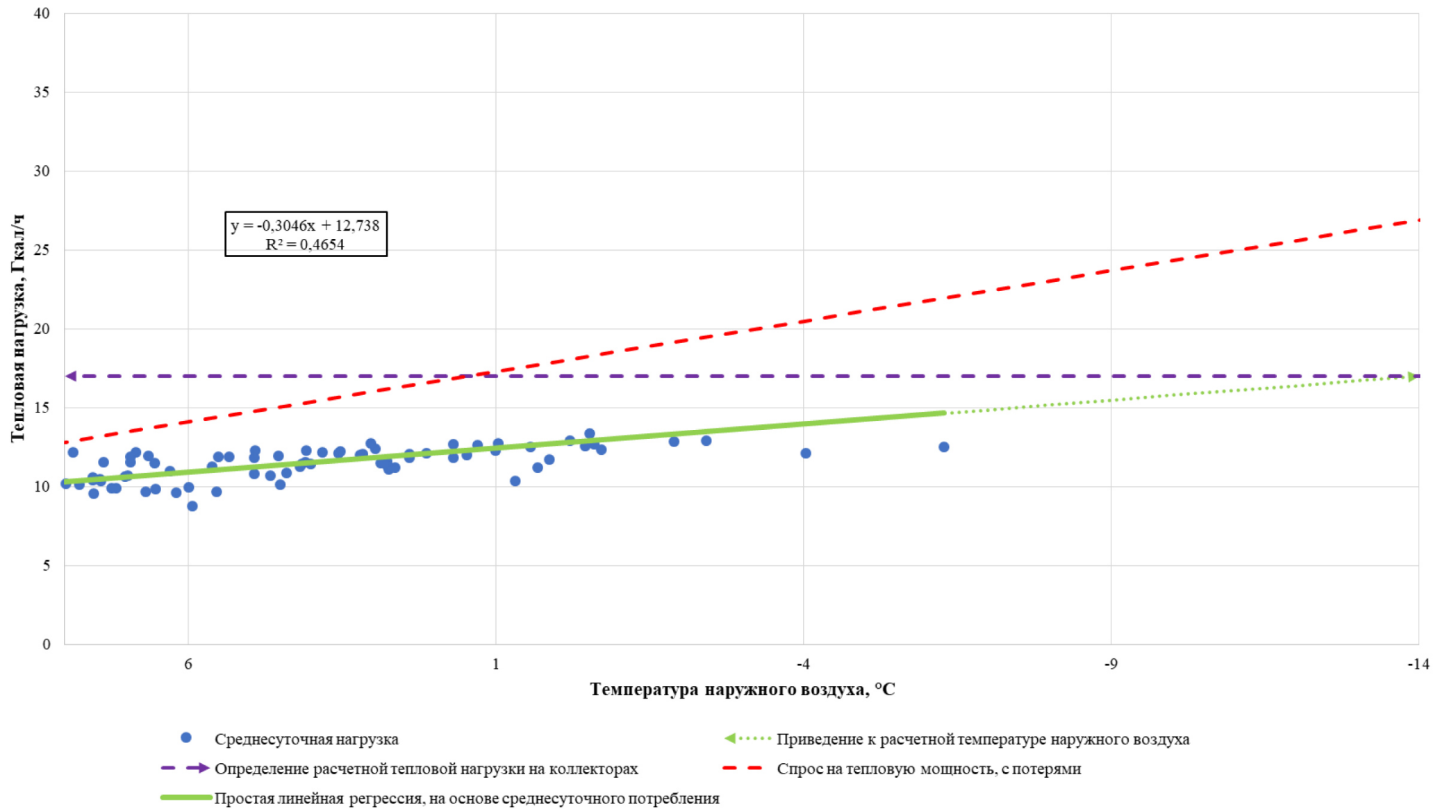
Рисунок 5.1 - Определение расчетной тепловой нагрузки на коллекторах в зоне действия котельной №1 АО «Теплоэнерго»
