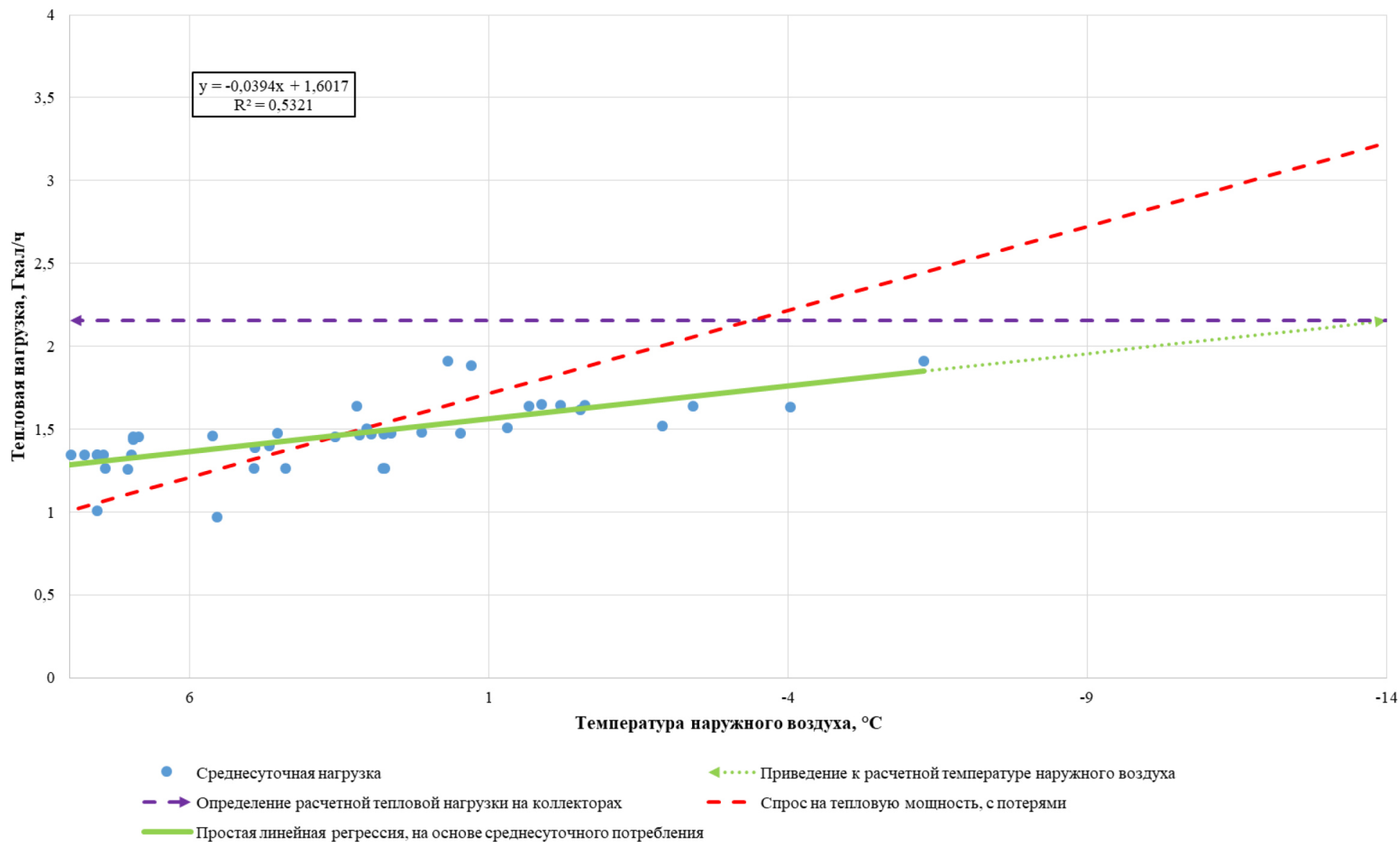
Рисунок 5.5 - Определение расчетной тепловой нагрузки на коллекторах в зоне действия котельной №6 АО «Теплоэнерго»
