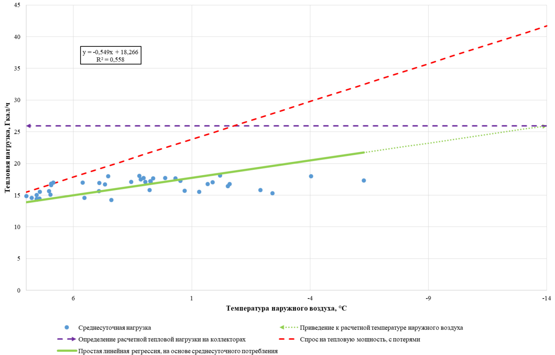
Рисунок 5.18 - Определение расчетной тепловой нагрузки на коллекторах в зоне действия котельной АО «Краснодартеплосеть»
