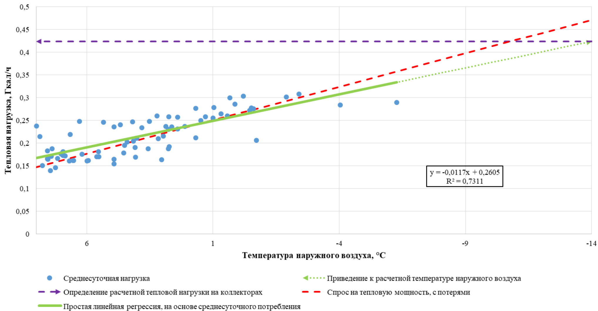
Рисунок 5.9 - Определение расчетной тепловой нагрузки на коллекторах в зоне действия котельной №10 АО «Теплоэнерго»
