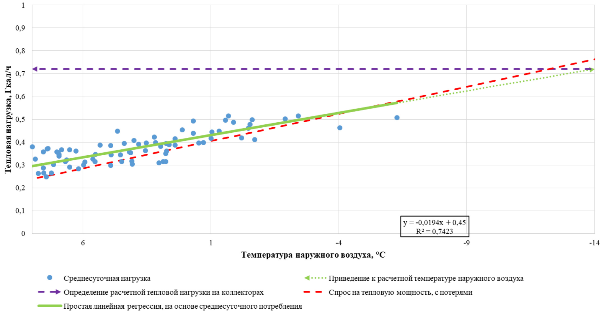
Рисунок 5.11 - Определение расчетной тепловой нагрузки на коллекторах в зоне действия котельной №14 АО «Теплоэнерго»
