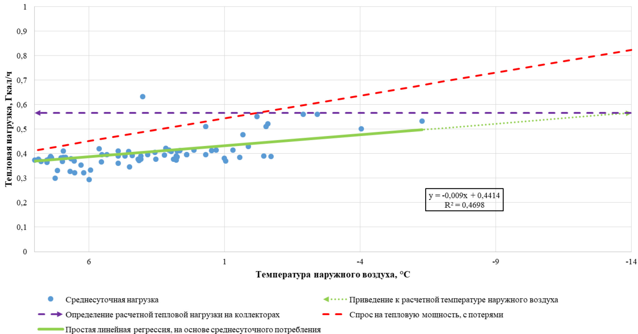
Рисунок 5.8 - Определение расчетной тепловой нагрузки на коллекторах в зоне действия котельной №9 АО «Теплоэнерго»
