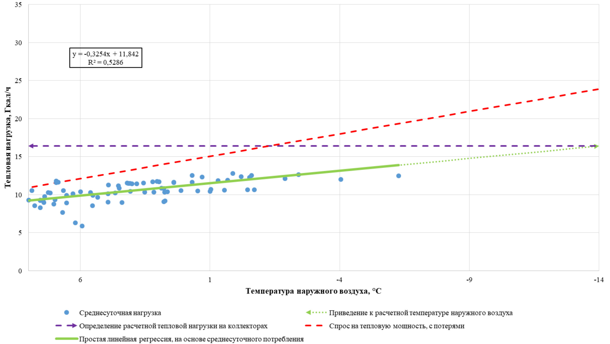
Рисунок 5.2 - Определение расчетной тепловой нагрузки на коллекторах в зоне действия котельной №2 АО «Теплоэнерго»
