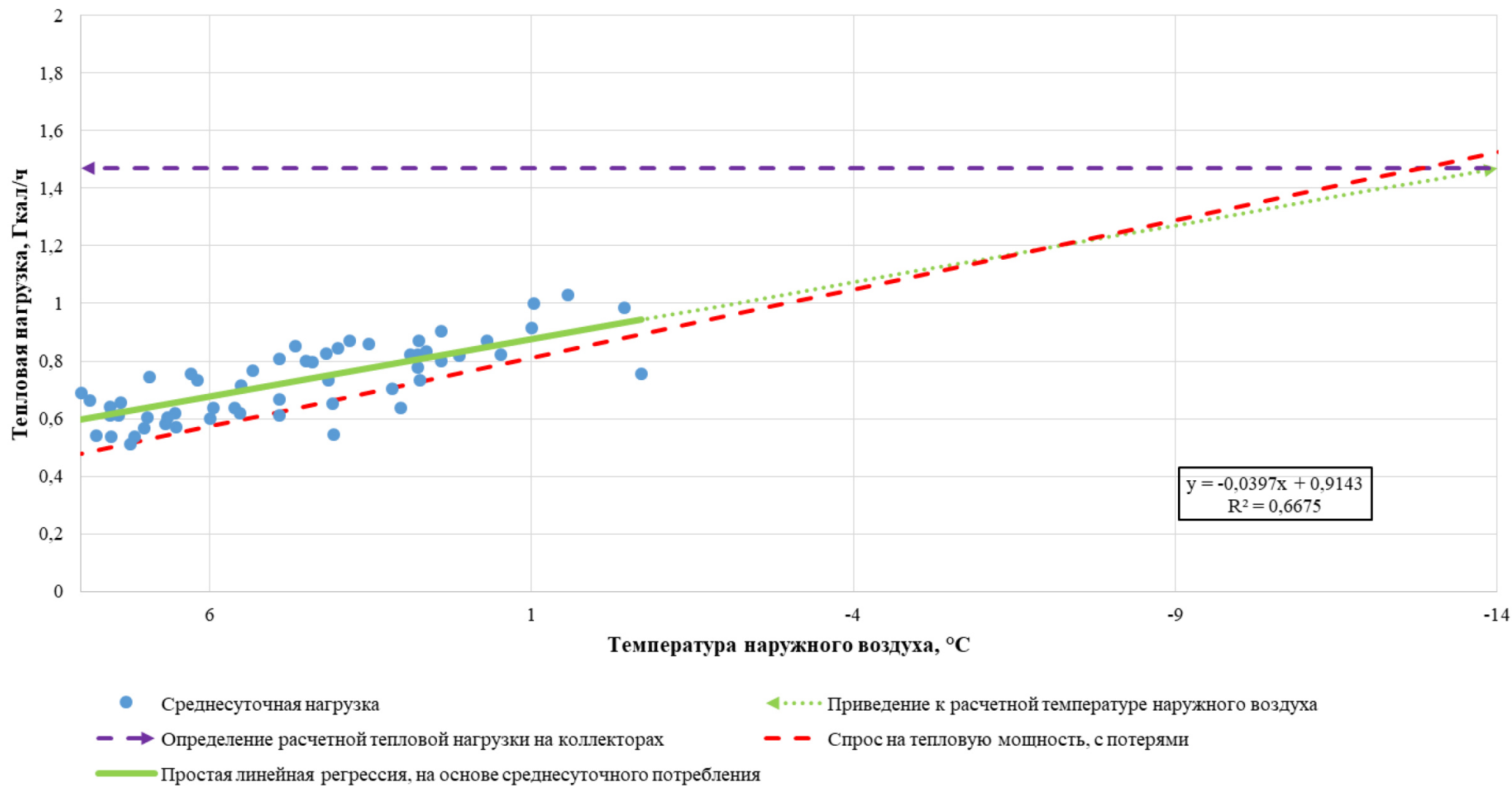
Рисунок 5.12 - Определение расчетной тепловой нагрузки на коллекторах в зоне действия котельной №16 АО «Теплоэнерго»
