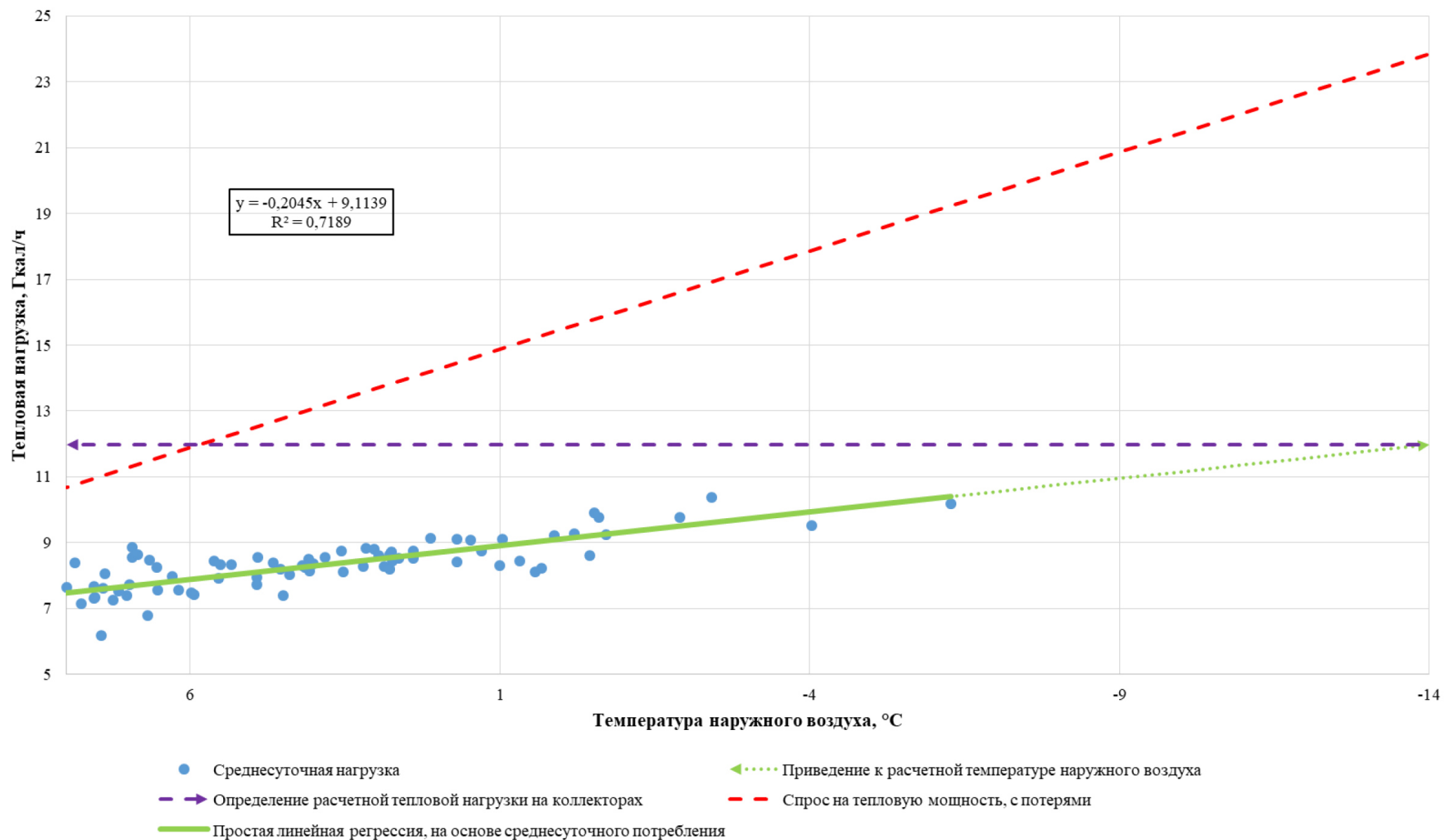
Рисунок 5.17 - Определение расчетной тепловой нагрузки на коллекторах в зоне действия котельной №3 ООО «Тепловик»
