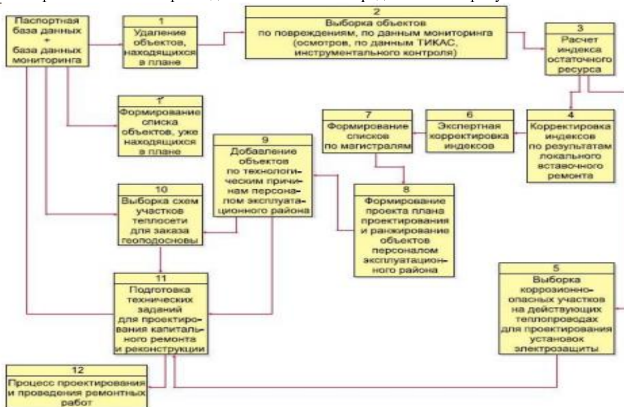
Рисунок 3.17 – Схема формирования плана проектирования и переключений
