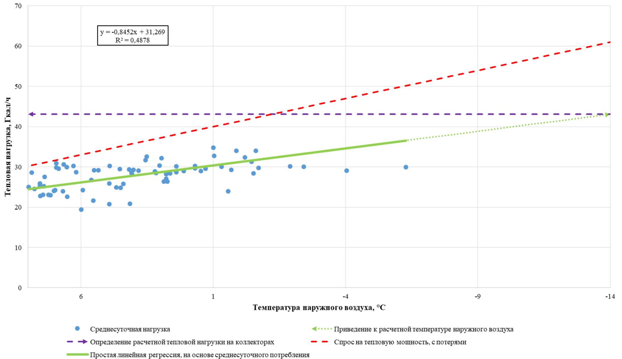
Рисунок 5.3 - Определение расчетной тепловой нагрузки на коллекторах в зоне действия котельной №3 АО «Теплоэнерго»
