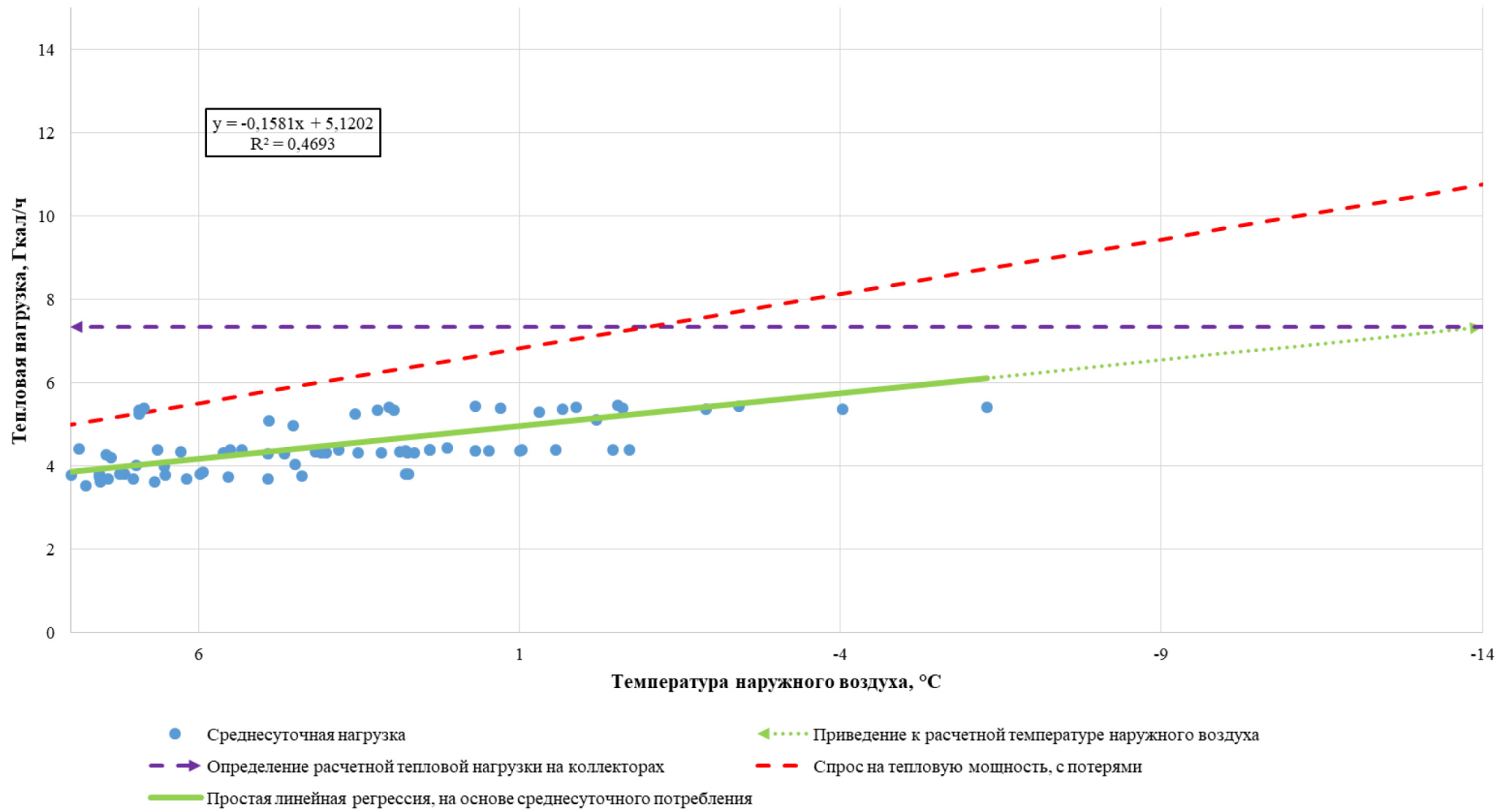
Рисунок 5.7 - Определение расчетной тепловой нагрузки на коллекторах в зоне действия котельной №8 АО «Теплоэнерго»
