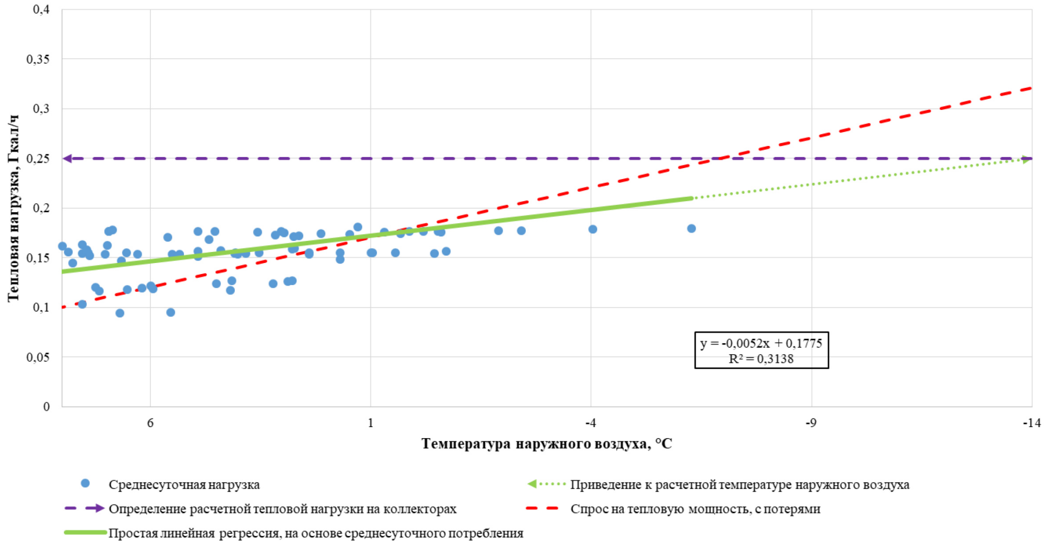
Рисунок 5.14 - Определение расчетной тепловой нагрузки на коллекторах в зоне действия котельной №21 АО «Теплоэнерго»
