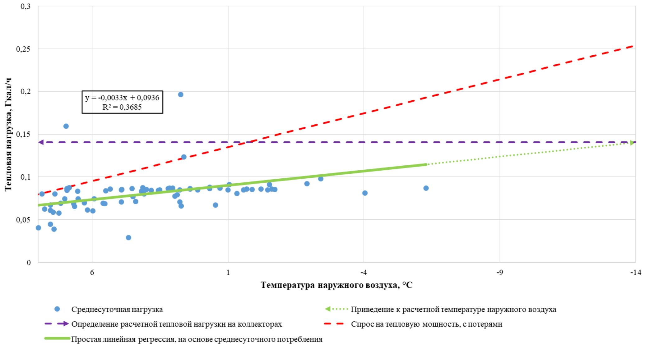
Рисунок 5.6 - Определение расчетной тепловой нагрузки на коллекторах в зоне действия котельной №7 АО «Теплоэнерго»
