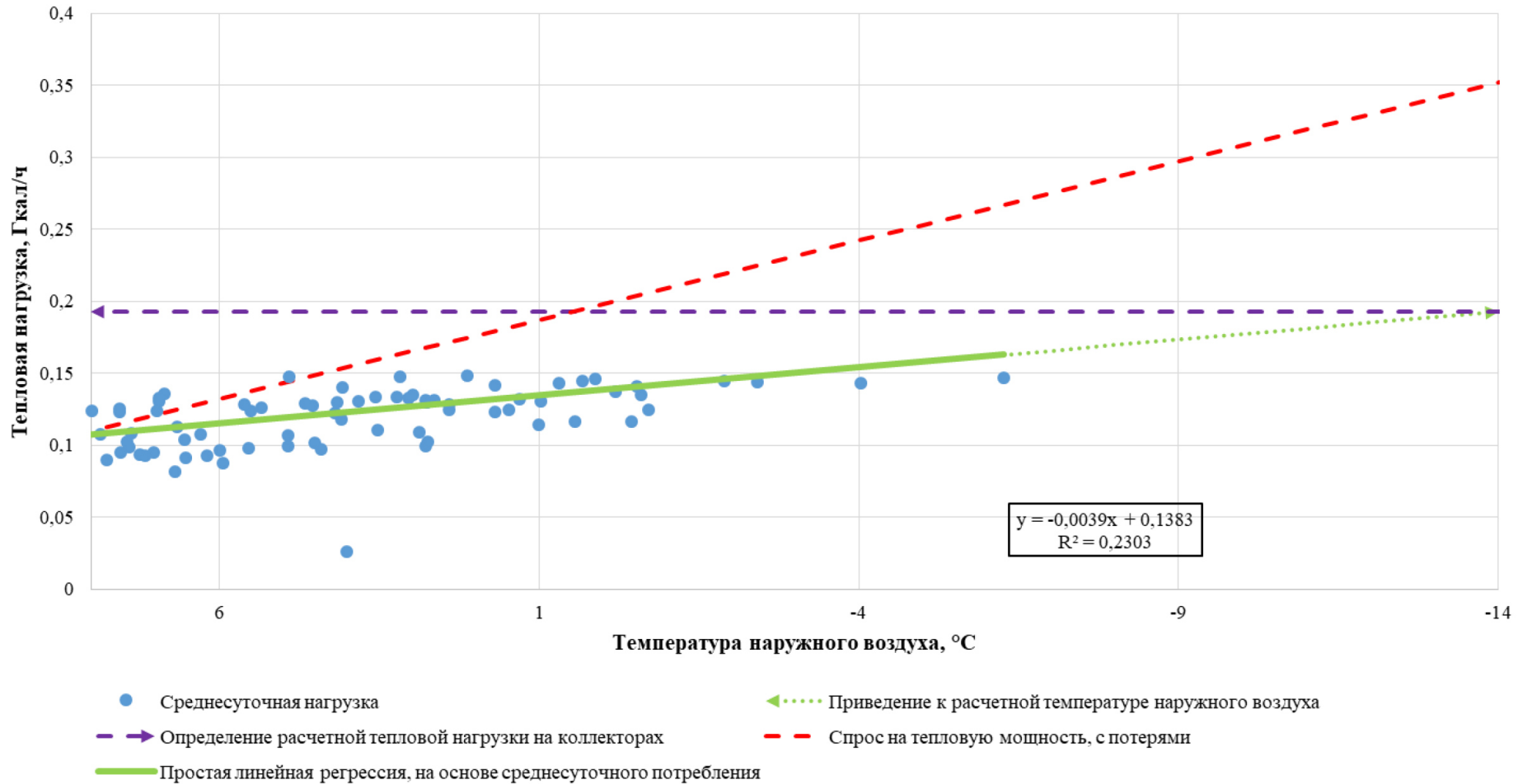
Рисунок 5.13 - Определение расчетной тепловой нагрузки на коллекторах в зоне действия котельной №20 АО «Теплоэнерго»
